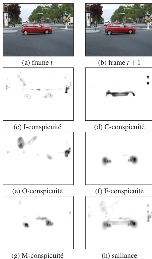
Figure 1: (c-g) Cartes de conspicuité calculées par [IDP03] à partir des frames (a-b). (h) carte de saillance calculée à partir de (c-g). Les régions saillantes apparaissent en noir.
